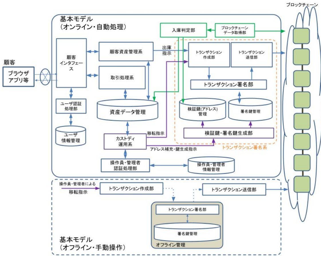
図7-1 署名鍵のオフライン管理のイメージ
